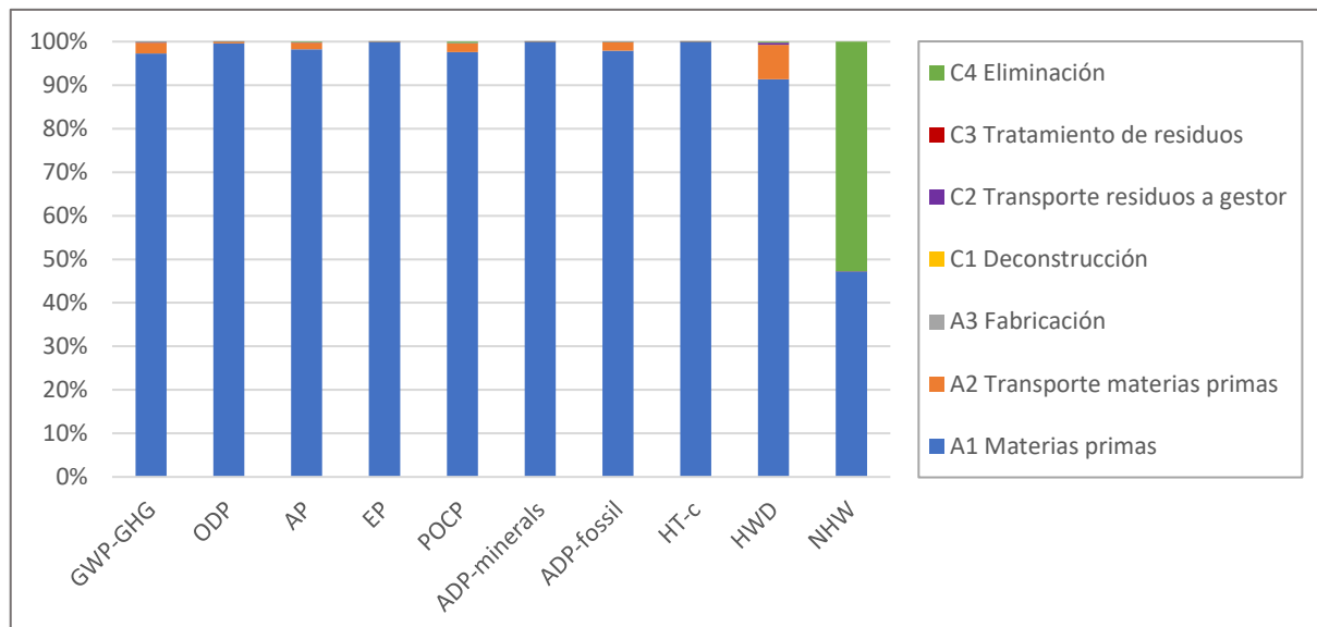
Contribución ambiental de los módulos del producto promedio representativo sobre su ciclo de vida
