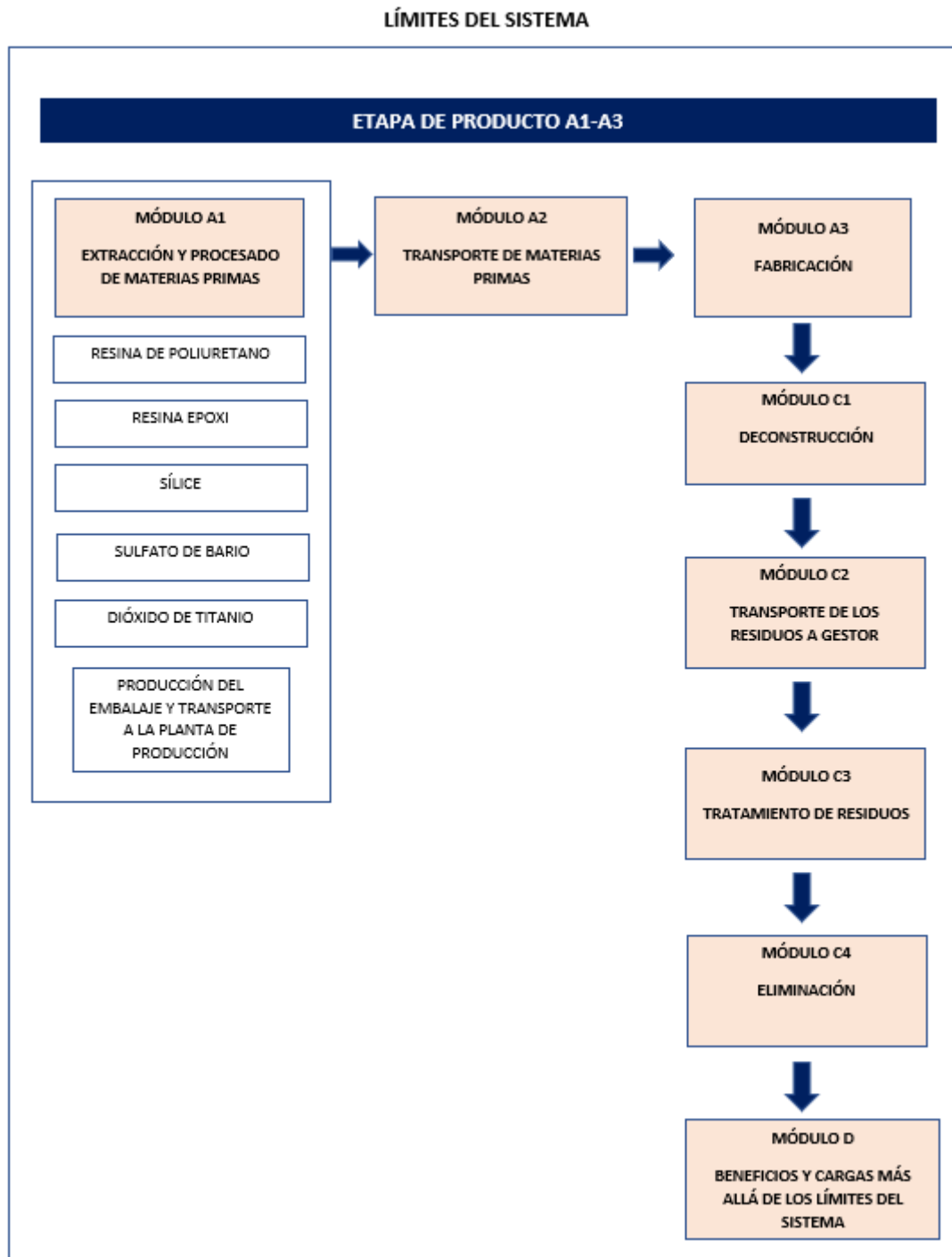
Ilustración 3. Diagrama de límites del sistema del producto
