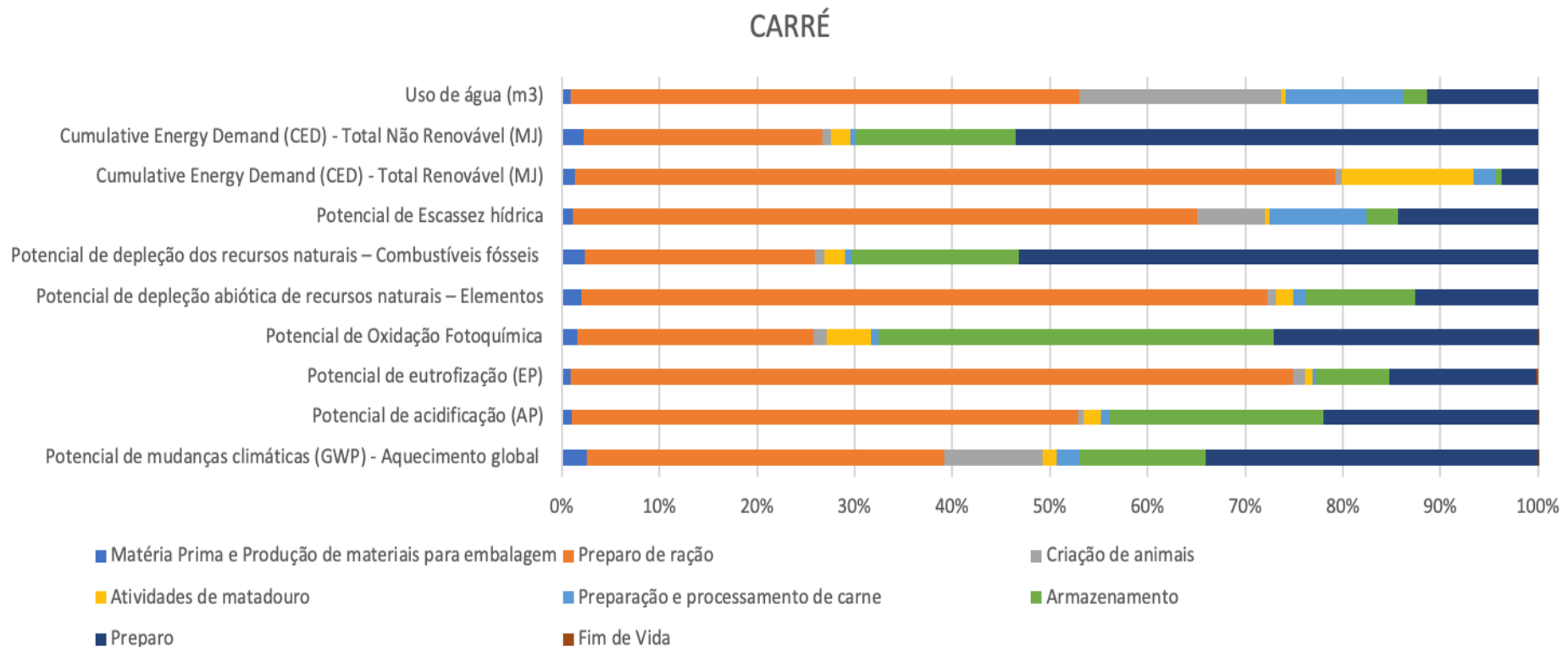
Gráfico 1 – Resultados das contribuições relativas das etapas do ciclo de vida para os potenciais impactos ambientais do carré
